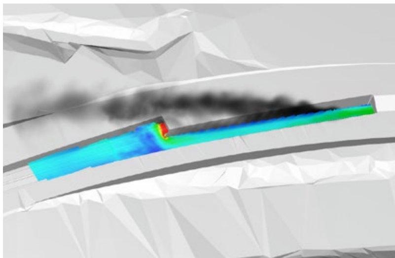
CFD-Brand- und Rauchausbreitungssimulationen
